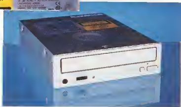
Seltsam, seltsam: In der Gehäuseabdeckung des ICD-3600/AT von Aztech befindet sich ein Loch für die Spindel des Motors. Hier darf nichts draufdrücken, sonst wird das Laufwerk gebremst.
